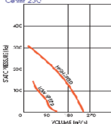
Centrif 250
